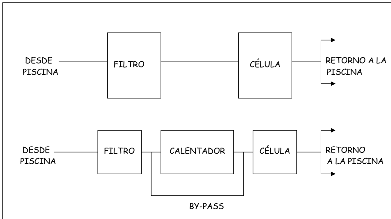
1 Esquema de montaje
