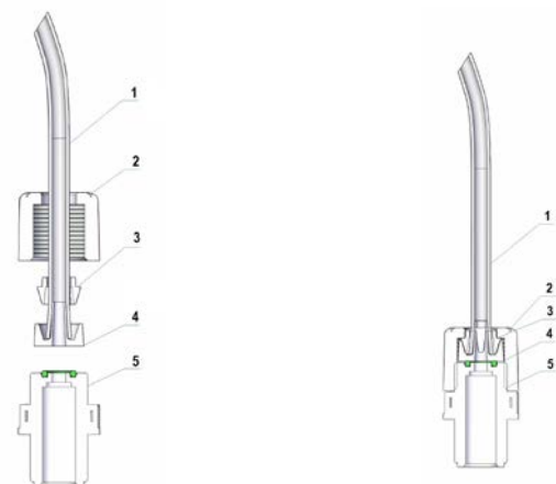
Fig.4 – Ligação hidráulica
