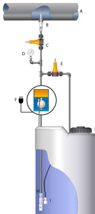
Fig. 6 – Impianto tipico
