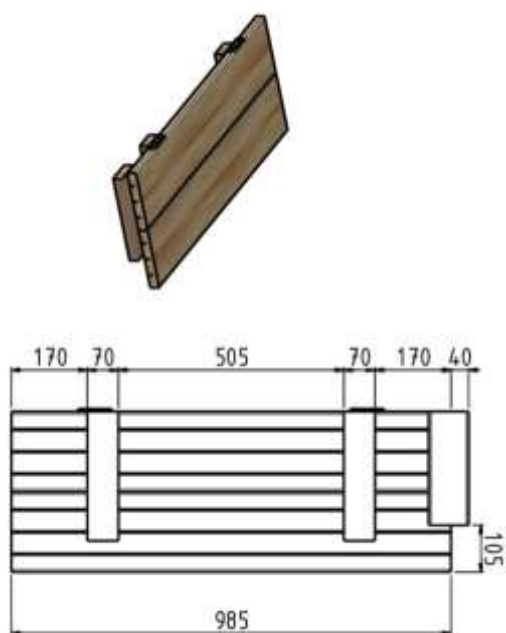
Figura 25 - Montaje de la rejilla de bloqueo
