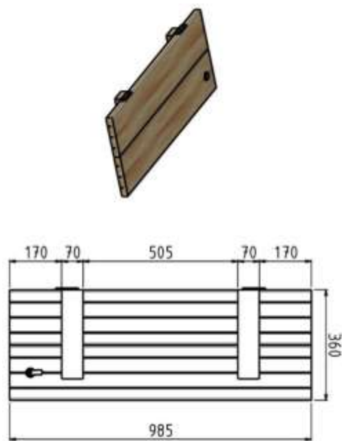
Figura 26 - Montaje de la rejilla con cerradura
