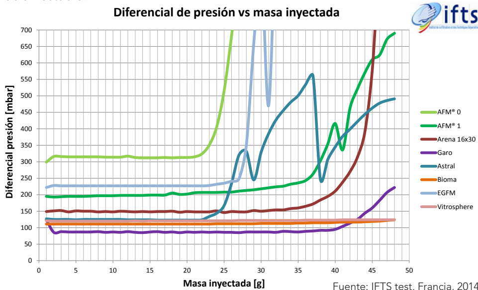
Gráfico 2: Diferencial de presión vs masa inyectada
